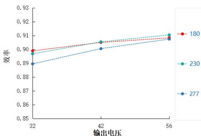
效率 VS 输出电压 HVE-75H-V56A/B
