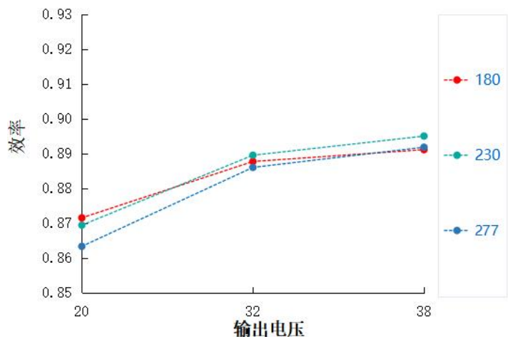
效率 VS 输出电压 HVE-75H-V38A/B
