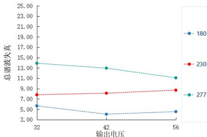
总谐波失真 VS 输出电压 HVE-75H-V56A/B
