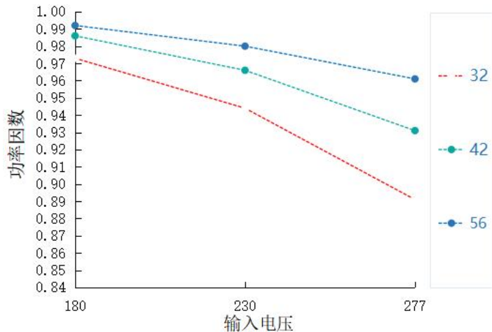
功率因素 VS 输入电压 HVE-75H-V56A/B
