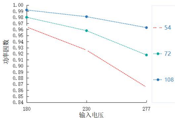
功率因素 VS 输入电压 HVE-75H-V108A/B
