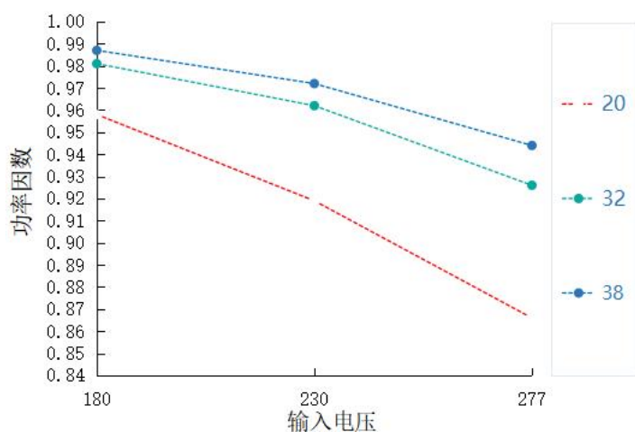
功率因素 VS 输入电压 HVE-75H-V38A/B
