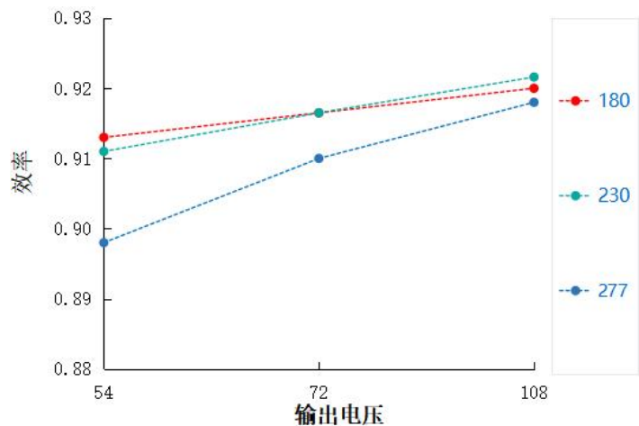
效率 VS 输出电压 HVE-75H-V108A/B
