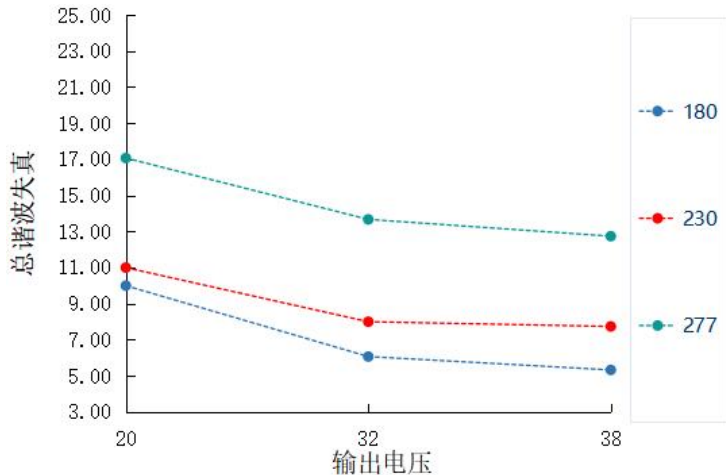
总谐波失真 VS 输出电压 HVE-75H-V38A/B
