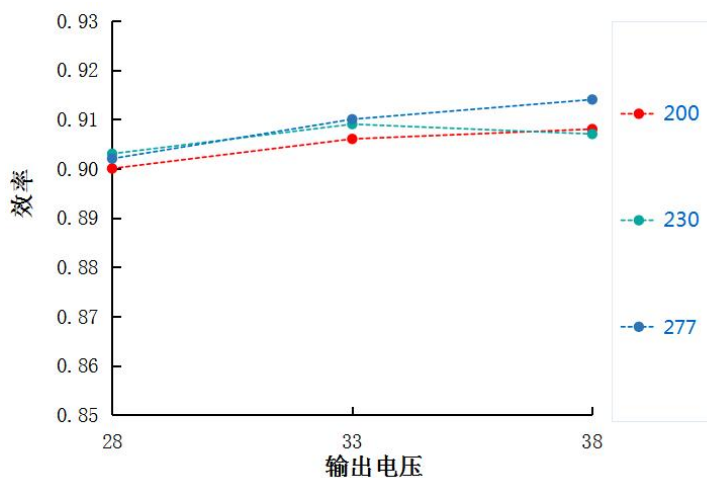
效率 VS 输出电压 HVE-143H-38A/B
