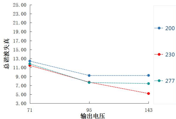
总谐波失真 VS 输出电压 HVE-100H-143A/B
