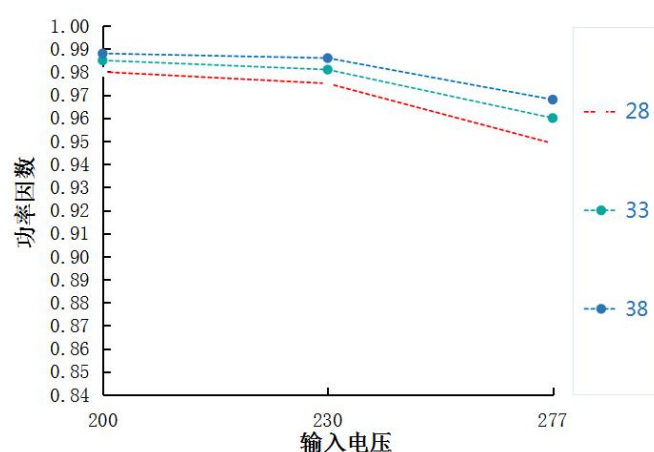
功率因素 VS 输入电压 HVE-100H-38A/B
