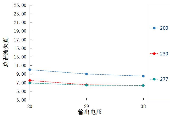
总谐波失真 VS 输出电压 HVE-100H-38A/B
