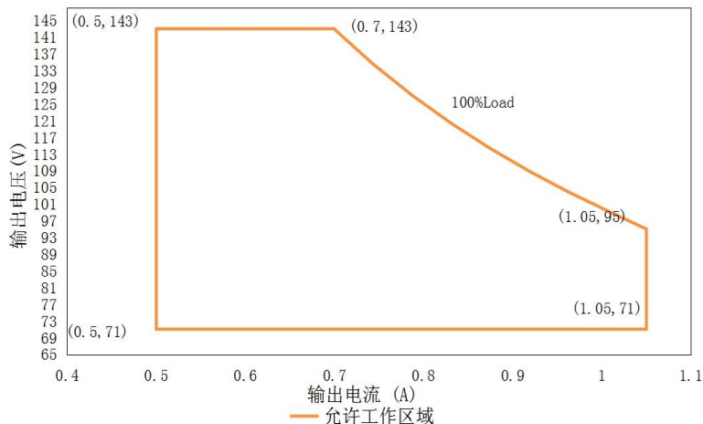
HVE-100H-143A/B (输入: 200-277Vac) 输出电压 VS 输出电流
