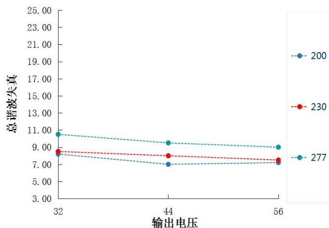
总谐波失真 VS 输出电压 HVE-100H-56A/B
