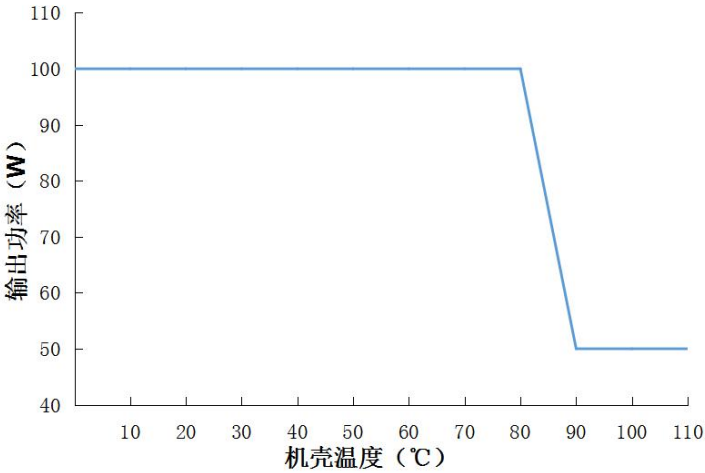
输出功率 VS 机壳温(HVE-100H-38/56/143A/B)
