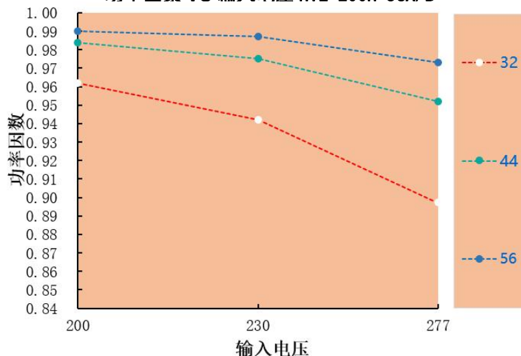
功率因素 VS 输入电压 HVE-200H-56A/B
