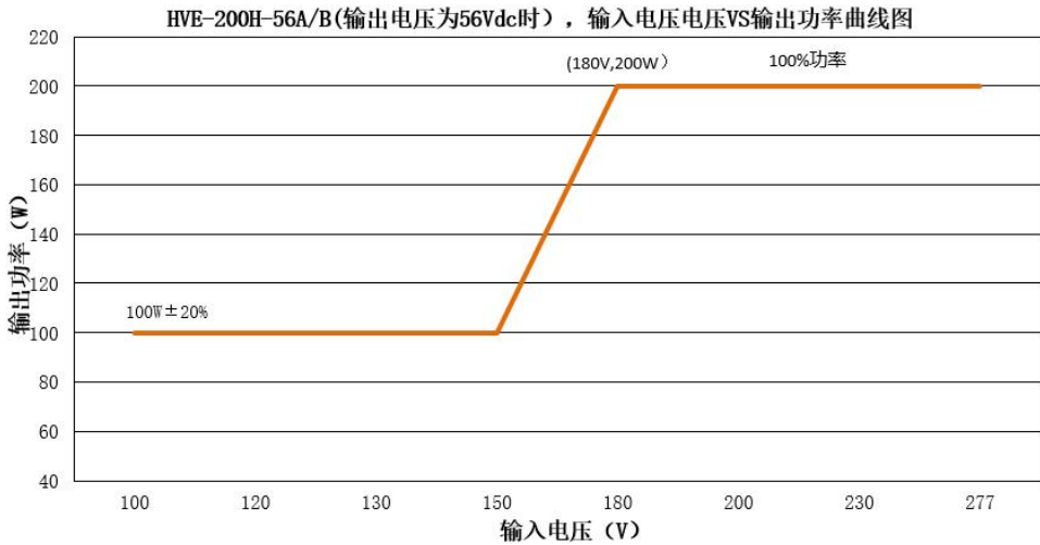
HVE-200H-56A/B(输出电压为 56Vdc 时，不同输入电压对应的额定输出电流值和输出功率)
