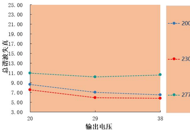
总谐波失真 VS 输出电压 HVE-200H-38A/B
