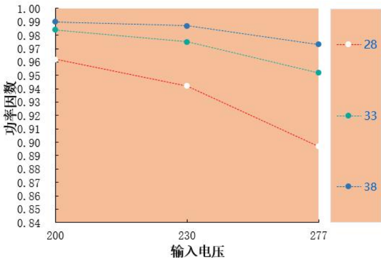
功率因素 VS 输入电压 HVE-200H-38A/B
