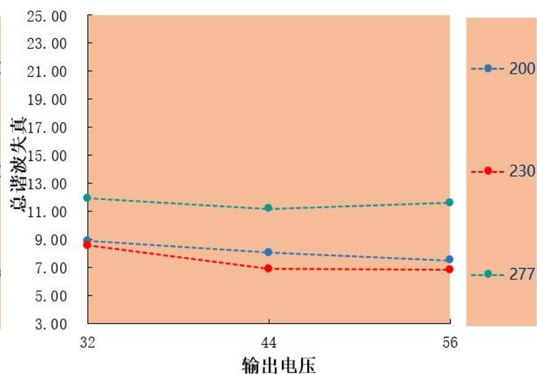
总谐波失真 VS 输出电压 HVE-200H-56A/B
