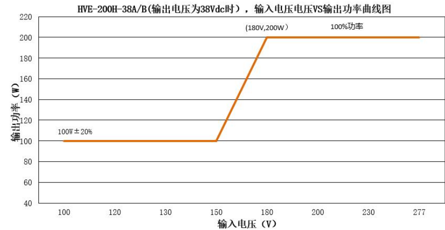
HVE-200H-38A/B (输出电压为 38Vdc 时，不同输入电压对应的额定输出电流值和输出功率)
