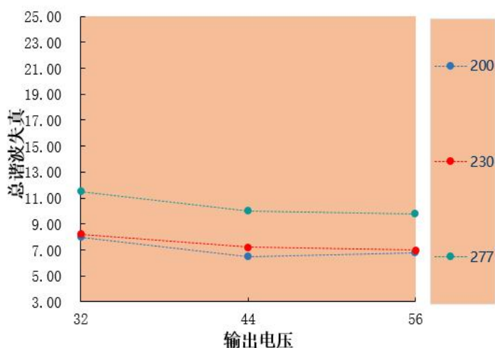
总谐波失真 VS 输出电压 HVE-240H-56A/B
