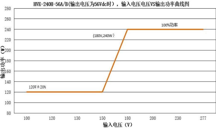
HVE-240H-56A/B(输出电压为 56Vdc 时，不同输入电压对应的额定输出电流值和输出功率)
