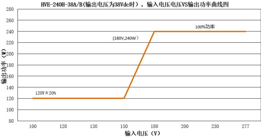
HVE-240H-38A/B (输出电压为 38Vdc 时，不同输入电压对应的额定输出电流值和输出功率)
