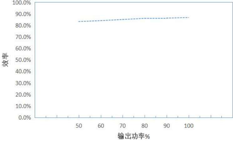
效率 VS 输出功率
