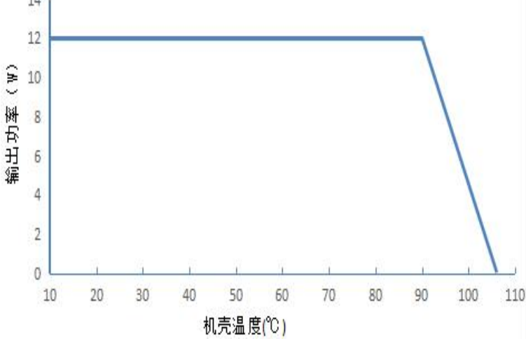
输出功率 VS 环境温度曲线
