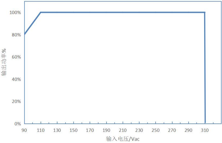
输出功率 VS 输入电压
