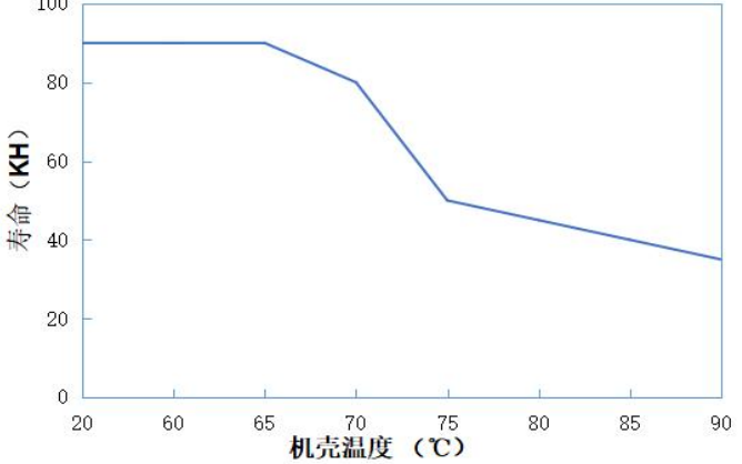
Tc VS 寿命 ( HAE-8W )
