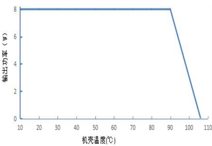
输出功率 VS 环境温度曲线
