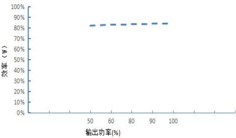
效率 VS 输出功率
