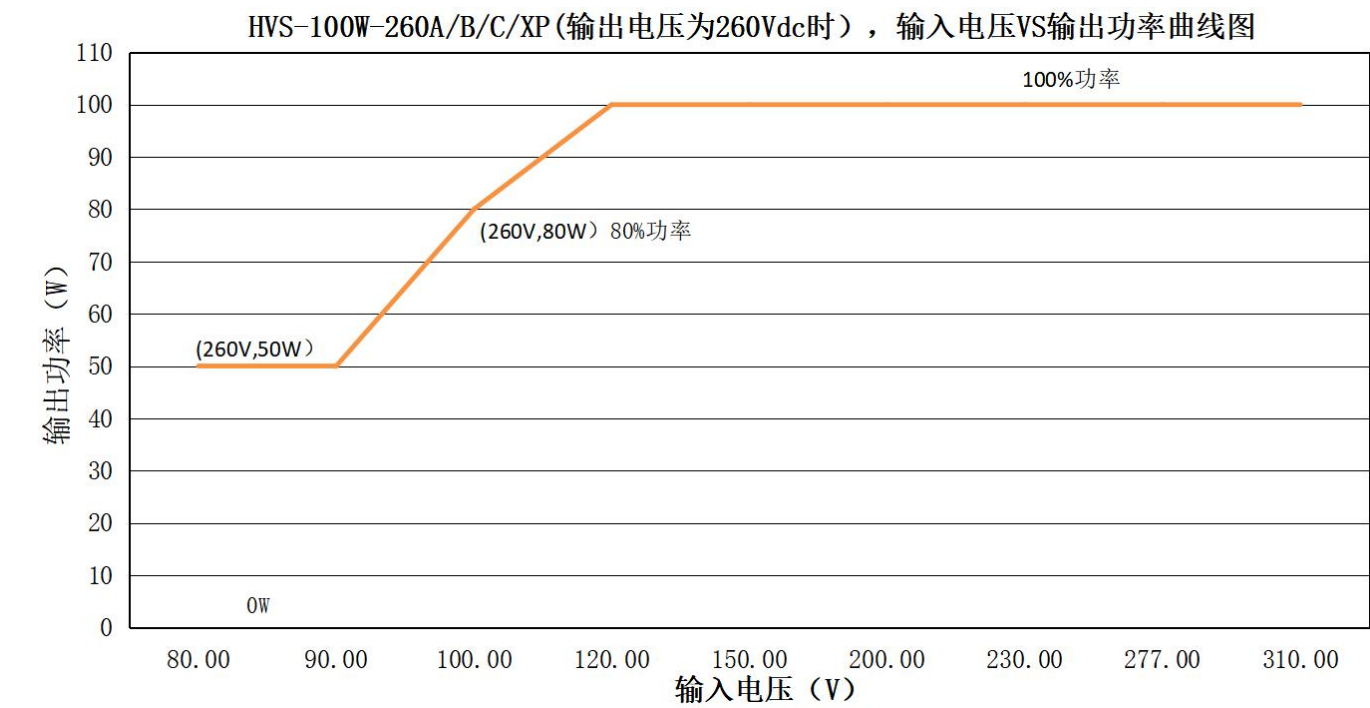
输出功率 VS 输入电压
