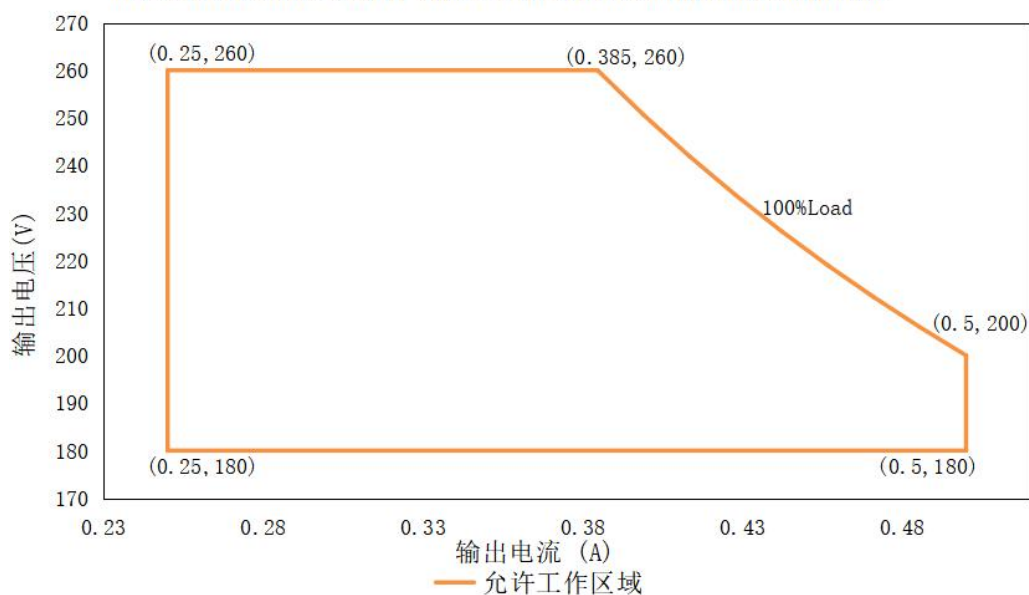
HVS-100W-260A/B/C/XP (输入: 100~277Vac) 输出电压VS输出电流
