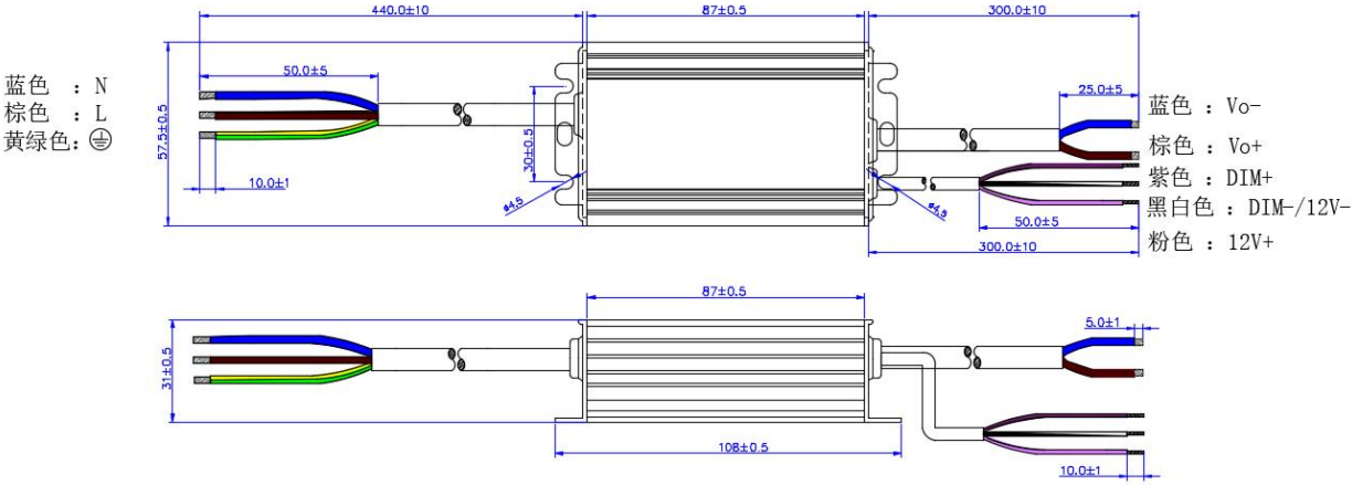
HVS-30W-150XP
