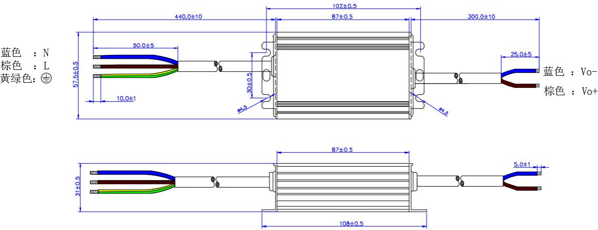
HVS-30W-150A
