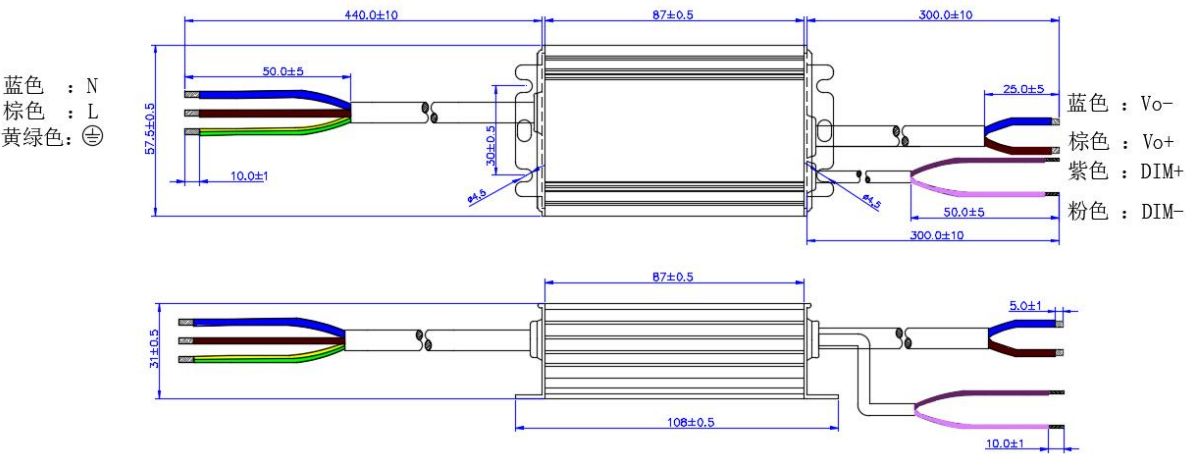
HVS-30W-150B
