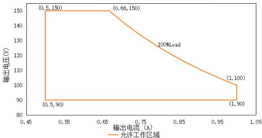
HVS-100W-150A/B/C (输入: 100-277Vac) 输出电压 VS 输出电流
