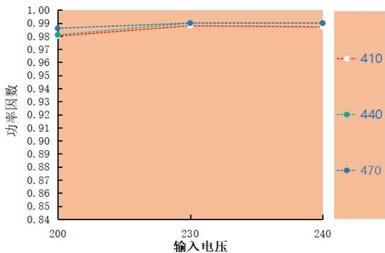
功率因素 VS 输入电压 LAS-100H-470A
