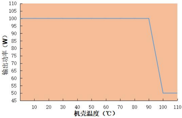
机壳温度 VS 输出功率 LAS-100H-470A-XP
