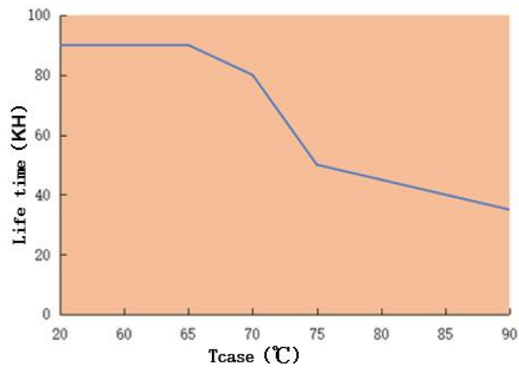
Tcase VS Life time LAG-50H-450A
