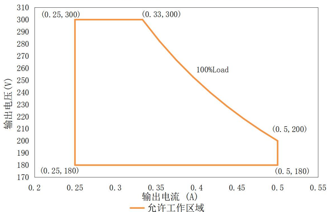
LCS-100W-300X (输入: 120-277Vac) 输出电压 VS 输出电流
