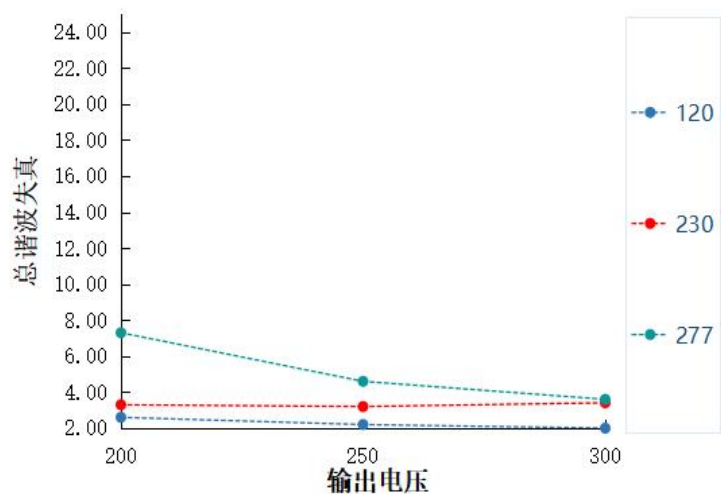
总谐波失真 VS 输出电压
