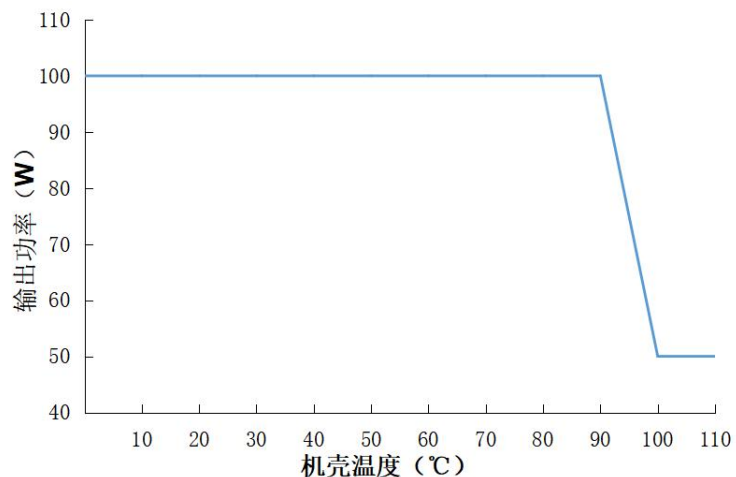
输出功率 VS 机壳温度
