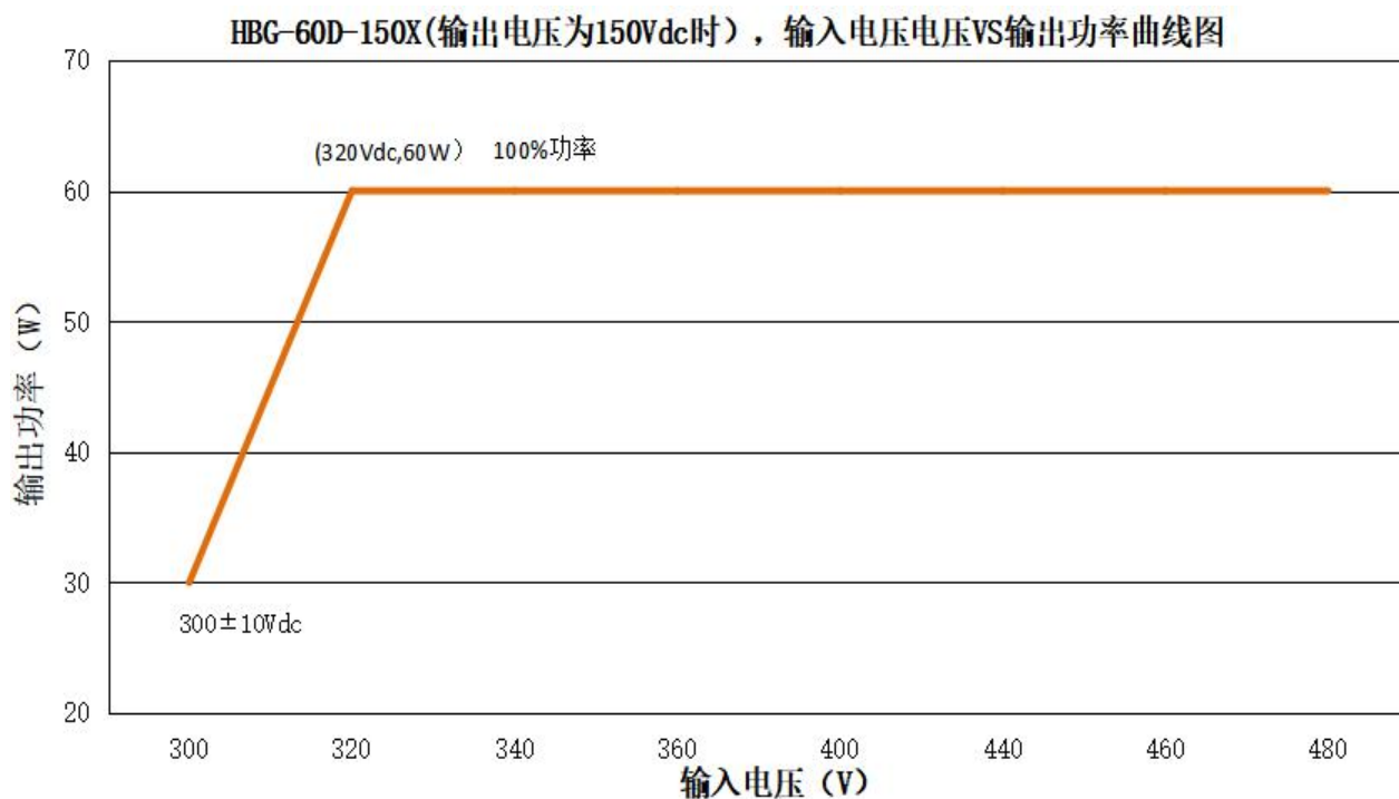
HBG-60D-150X (输出电压为 150Vdc 时，不同输入电压对应的额定输出电流值和输出功率)
