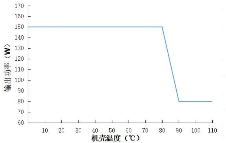
输出功率 VS 机壳温(HBG-150D-150A/P)
