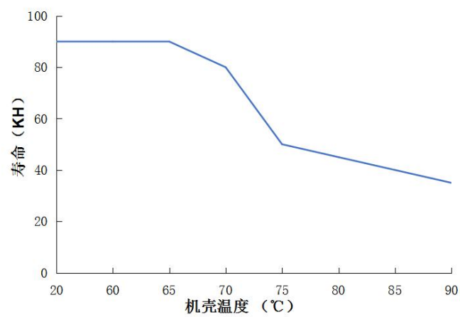
Tc VS 寿命(HBG-150D-150A/P)
